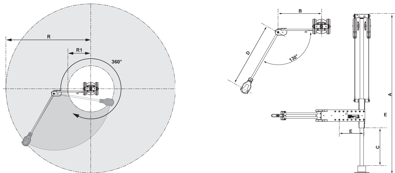
Характеристики линейной штанги D53 с указанием охватываемого рабочего пространства
