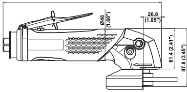
KA16135C4FK = 238 мм (9.37")
