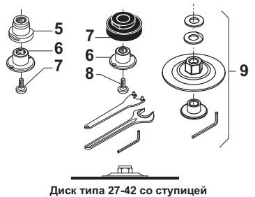
Диск типа 27-42 со ступицей
