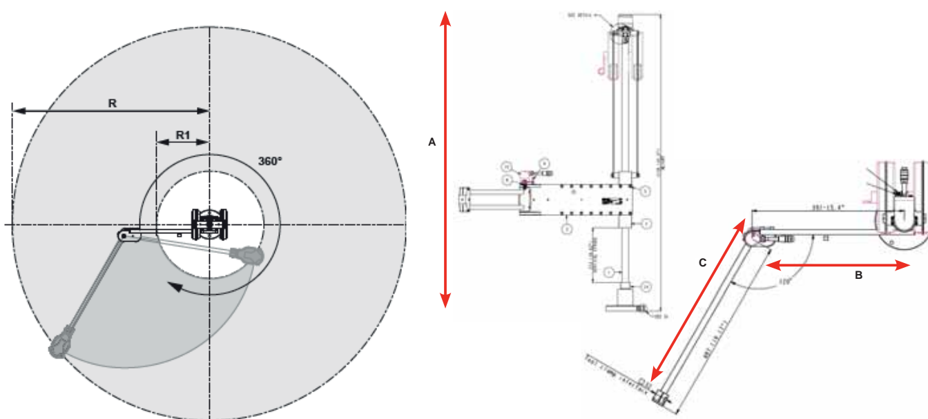
Складная штанга
