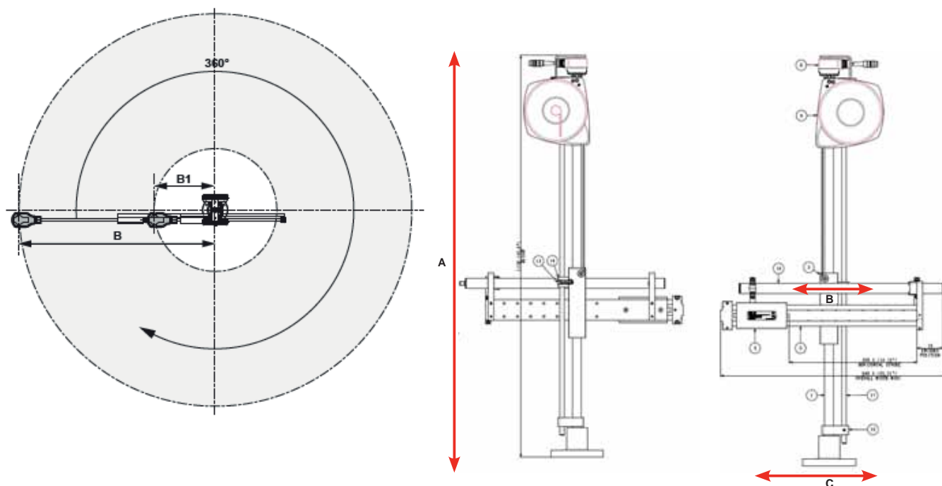
Линейная штанга
